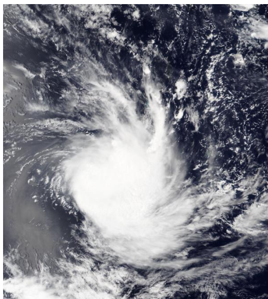
Passage du Cyclone BELAL à La Réunion, janvier 2024. Source: Worldview: Explore Your Dynamic Planet, 2024 (N.A.S.A.)
